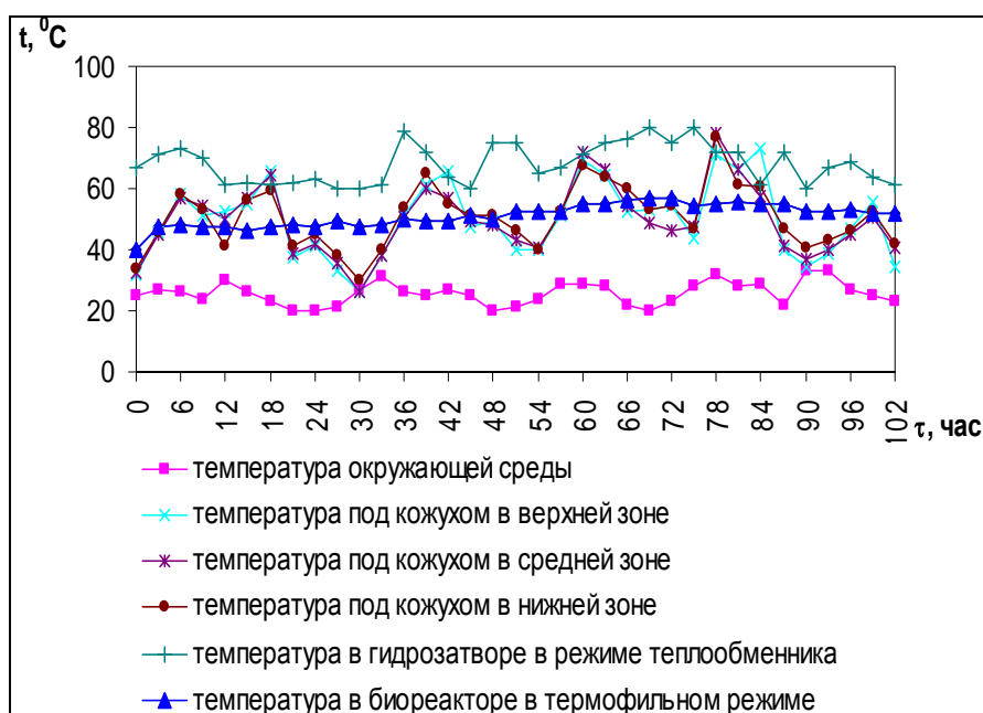
Рисунок 2 – Зависимости параметров метантенка от времени при нагреве в термофильном режиме
